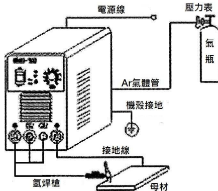
氬焊接線圖
