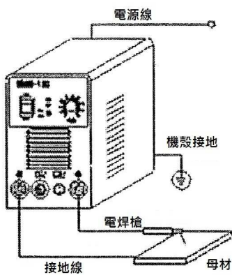
電焊接線圖
