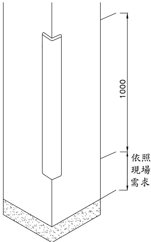
柱角防護條施工位置圖
