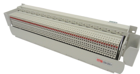
23" 145mm 64-circuit E1 DDF
