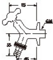
34-205 庭院古典水栓(插管接頭) 古絲
