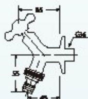
34-203 庭院古典水栓(快速接頭) 古絲
