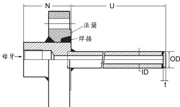
牙口套管
