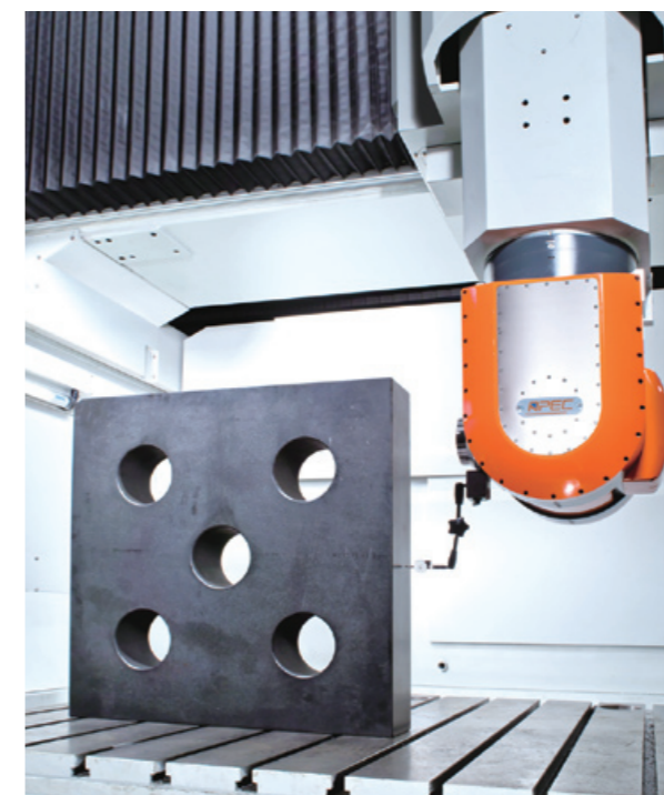
1m X 1m 花崗岩幾何精度測試確保 XY、XZ、與 YZ 之空間幾何精度
